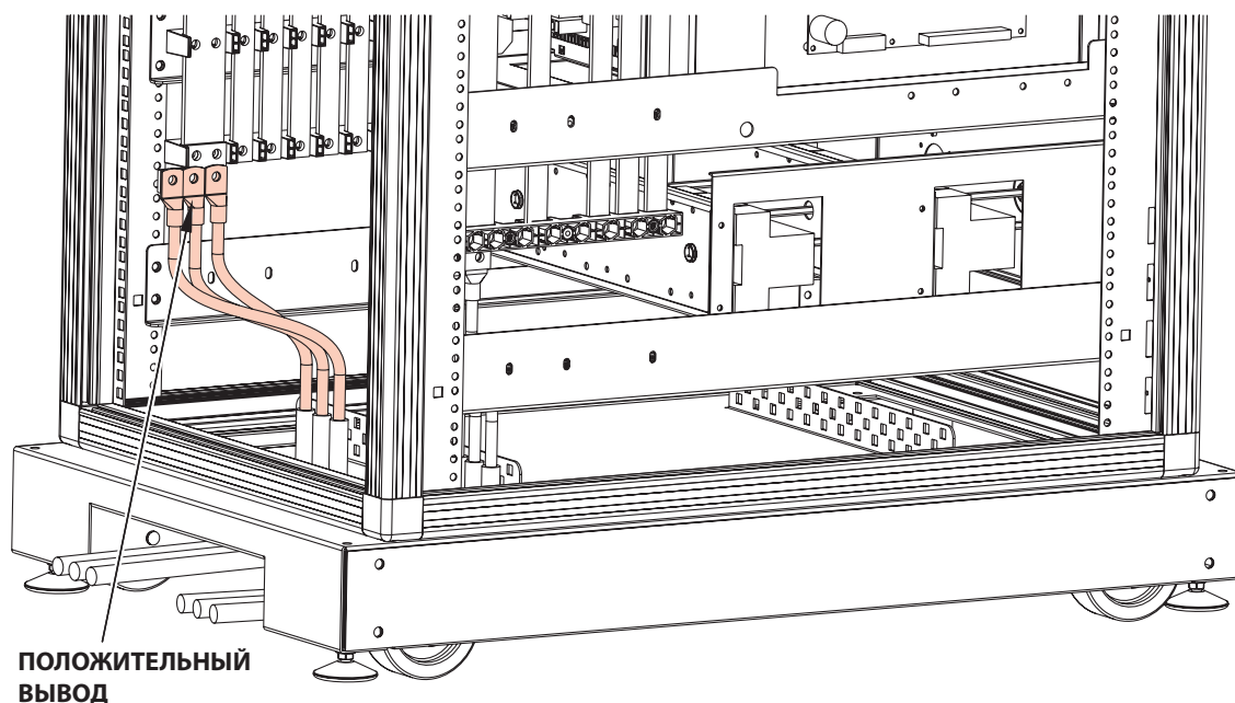
Подключение внешних батарейных кабинетов Archimod® 80-100-120 кВА – вид сзади, положительный полюс
