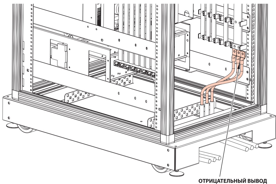
Подключение внешних батарейных кабинетов Archimod® 80-100-120 кВА – вид сзади, отрицательный полюс
