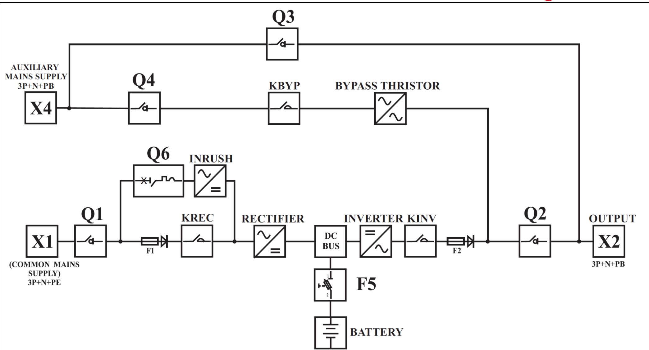
СХЕМА ОДИНОЧНОГО ИБП С РАЗДЕЛЬНЫМИ ВВОДАМИ ВЫПРЯМИТЕЛЯ И БАЙПАСА (80-120 кВА)
