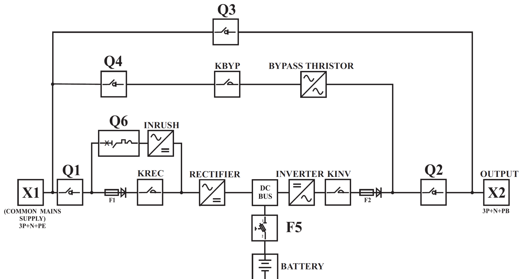
СХЕМА ОДИНОЧНОГО ИБП С ОБЩИМ ВВОДОМ ВЫПРЯМИТЕЛЯ И БАЙПАСА (80-120 кВА)
