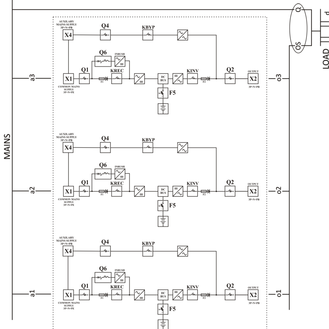
Конфигурация N+1 с тремя параллельными ИБП (80-120 кВА) и одним вводом от распределительного устройства
