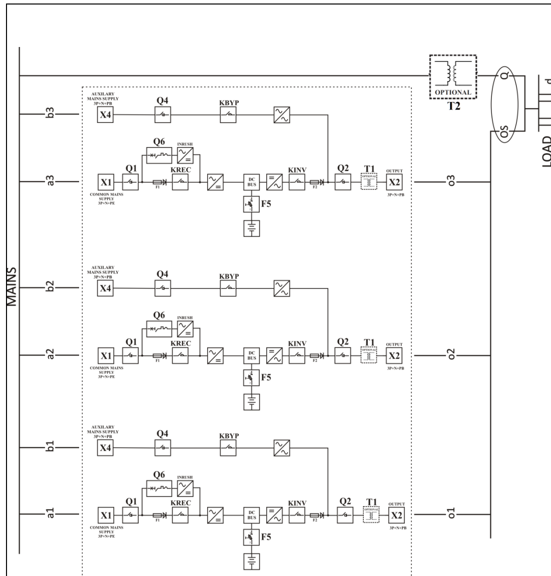
Конфигурация N+1 с тремя параллельными ИБП (10-60 кВА) и двумя вводами от распределительного устройства
