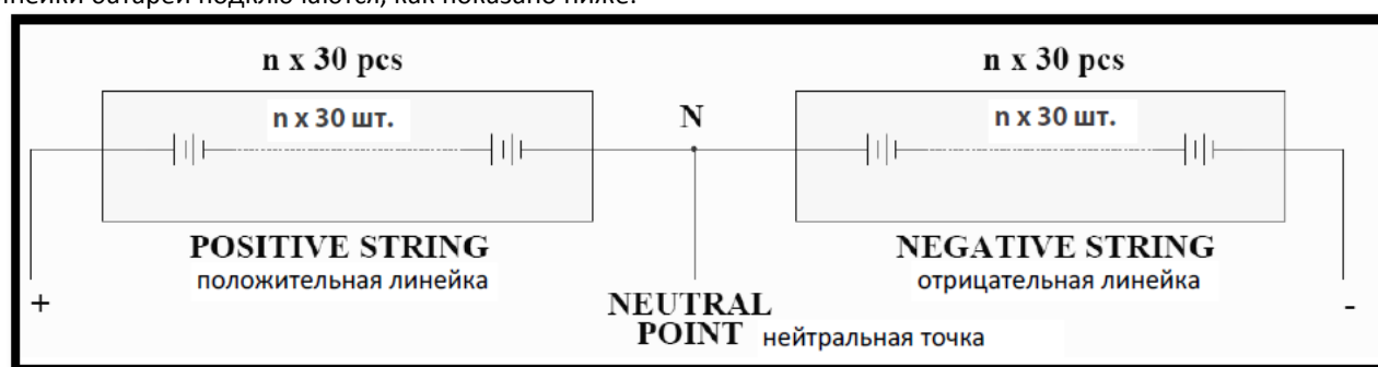
Две линейки аккумуляторов и нейтральная точка
